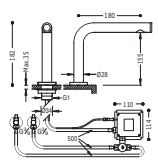
Lavabo electrónico mezclador TOUCH-TRES Sistema sensible al tacto. Sólo tocar (NO pulsar). NOTA: Incluye un grifo mezclador dos aguas con tubos flexibles (ref. 1.92.507.30).
