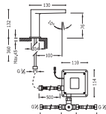
Lavabo electrónico mezclador Accionado mediante sensor de infrarrojos. NOTA: Incluye un grifo mezclador dos aguas con tubos flexibles (ref:1.92.507.30).
