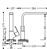
Monomando fregadero vertical caño de 35x15 mm.
