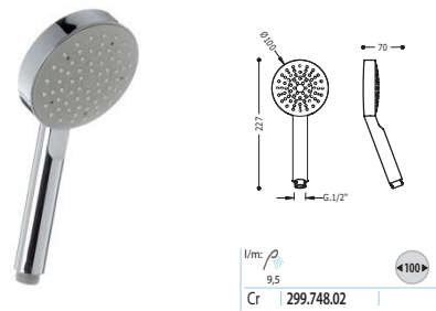
Ducha anticalcárea PAUSA
