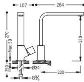
Monomando fregadero vertical caño de 35x15 mm.
