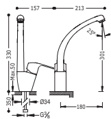
Monomando fregadero vertical
