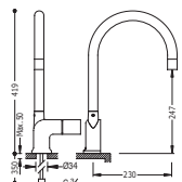
Monomando fregadero vertical con rociador extraíble
