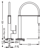
Monomando fregadero vertical con rociador extraíble
