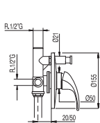
Monomando empotrar (2 vías) cuerpo empotrado incluido
