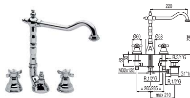
Batería lavabo De instalación libre.
