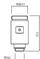
Válvula de vaciado LEX, MAX Anterior 2012 (para ref.: 81.385, 81.191)
