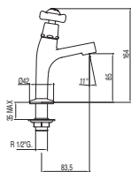
Grifo lavabo 1 agua o premezclada
