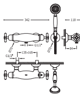
Ducha termostática Ducha de mano anticálcarea con soporte orientable. Flexo doble engatillado
