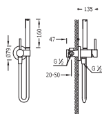
Monomando empotrar para bidé WC
