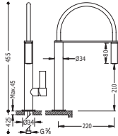
Monomando fregadero vertical con rociador extraíble
