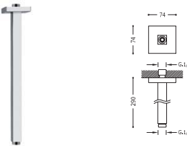
Brazo techo para rociador ducha
