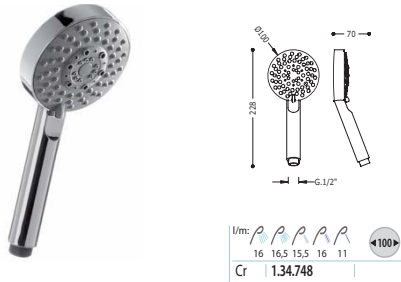
Ducha masaje PAUSA
