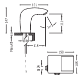
Lavabo electrónico 1 agua Accionado mediante sensor de infrarrojos
