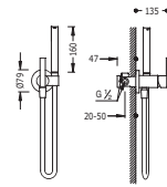
Monomando mezclador empotrar para bidé WC
