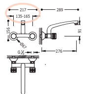
Grupo fregadero pared
