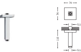
Brazo techo para rociador ducha
