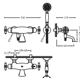
Bañera-ducha termostática Ducha de mano anticálcarea con soporte orientable. Flexo doble engatillado
