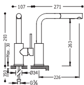
Monomando fregadero vertical con ducha extraíble.
