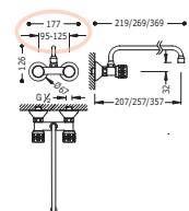
Grupo fregadero pared
