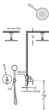
Kit de ducha monomando empotrado con cierre y regulación de caudal. - Cuerpo empotrado incluido - Ducha fija Ø 225 mm. con rótula. (299.632.01). - Soporte con toma pared (205.182.01). - Ducha anticalcárea Ø 100 mm. - Flexo SATIN (91.34.609.15).
