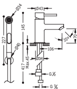
Monomando lavabo para bidé WC Duchita con cierre y flexo SATIN
