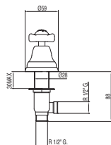
Grifo lateral batería lavabo
