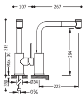
Monomando fregadero vertical con ducha extraíble (2 funciones)
