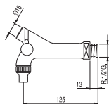
Grifo de vino Nº 2/N
