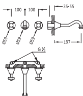
Batería lavabo mural Cuerpo empotrado incluido e indivisible.
