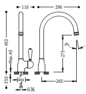
Monomando fregadera vertical con rociador extraíble
