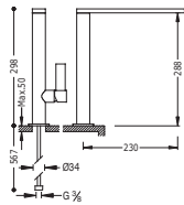
Monomando fregadero vertical caño de 34x9 mm.
