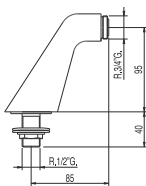
Codo adaptador baño-ducha 2 unidades con silenciador
