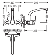
Monomando fregadero pared
