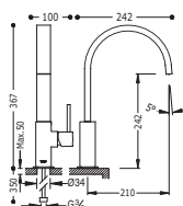
Monomando fregadero vertical caño 35x15 mm. con aireador rectangular oculto
