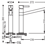
Monomando fregadero vertical caño largo
