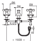
Batería bidé con duchita
