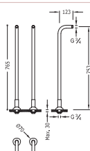
Tomas de agua a suelo de bañera 2 unidades
