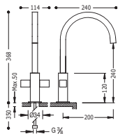
Bimando fregadero vertical caño de 22x22 mm.
