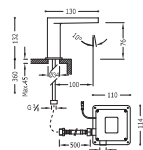
Lavabo electrónico 1 agua Accionado mediante sensor de infrarrojos
