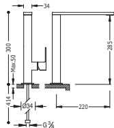
Monomando fregadero vertical caño de 34x10 mm.
