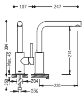
Monomando fregadero vertical
