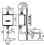
Grifo electrónico empotrado para urinario
