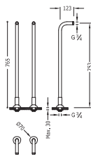
Tomas de agua a suelo de bañera 2 unidades
