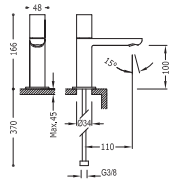
Monomando lavabo de repisa
