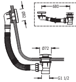
Desagüe bañera con rebosadero Tapón Ø 72 mm CLICK-CLACK
