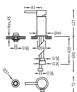
Monomando bidé con ducha
