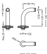
Codo adaptador baño-ducha 2 unidades con silenciador
