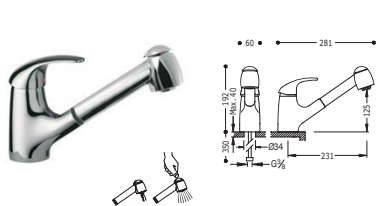
Monomando fregadero vertical con ducha extraíble (2 funciones)
