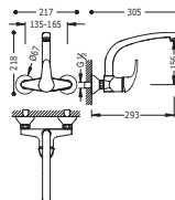
Monomando fregadero pared
