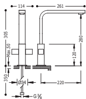
Bimando fregadero vertical caño de 35x15 mm.
