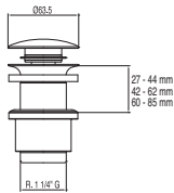
Válvula ciega para lavabo de madera Tapón Ø 63,5 mm CLICK-CLACK
