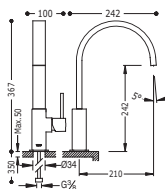
Monomando fregadero vertical caño 35x15 mm. con aireador rectangular oculto
