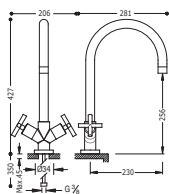
Bimando fregadero vertical
