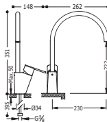
Monomando fregadero vertical
