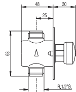
Grifo de urinario para empotrar rosca macho 1/2" G.
