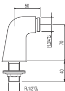
Codo adaptador baño-ducha 2 unidades con silenciador
