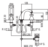
Batería lavabo De instalación libre.
