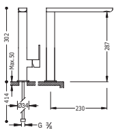
Monomando fregadero vertical caño de 34x15 mm.
