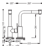
Monomando fregadero vertical con ducha extraíble (2 funciones)
