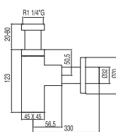
Sifón lavabo visto cuadrado telescópico
