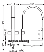
Bimando fregadero vertical caño 35x15 mm. con aireador rectangular oculto
