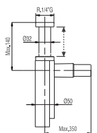
Sifón lavabo visto telescópico con faldón
