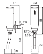
Grifo electrónico visto para urinario Con dos tubos adaptables a urinario
