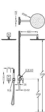
Kit de ducha monomando empotrado
