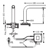
Lavabo electrónico 1 agua TOUCH-TRES Sistema sensible al tacto. Sólo tocar (NO pulsar)
