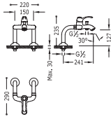
Monomando bañera de repisa Ducha de mano anticálcarea. Flexo doble engatillado
