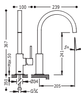
Monomando fregadero vertical caño de 22x22 mm.
