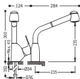
Monomando fregadero vertical con ducha extraíble (2 funciones)
